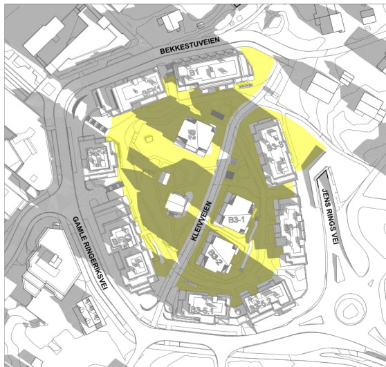
MUA - Sol/skyggediagram 21.03 - kl. 09:00
