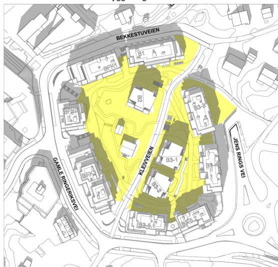
MUA - Sol/skyggediagram 21.03 - kl. 13:00
