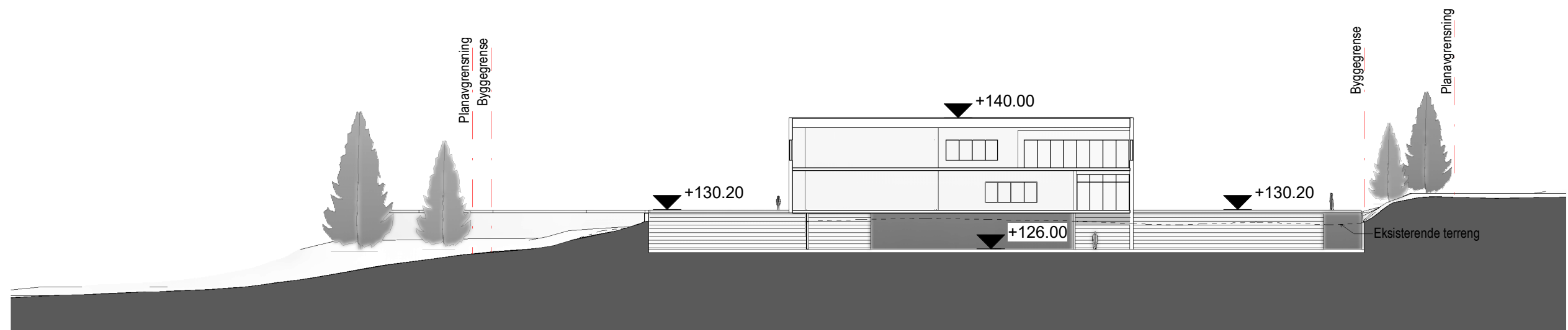
Prinsippsnitt øst-vest 1 : 500
