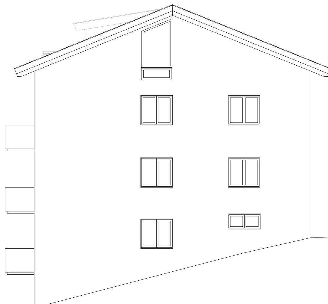
FASADE NORDØST
