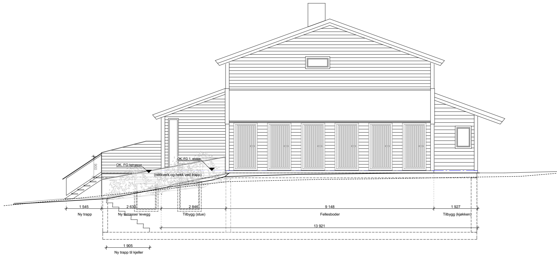
Fasade syd
