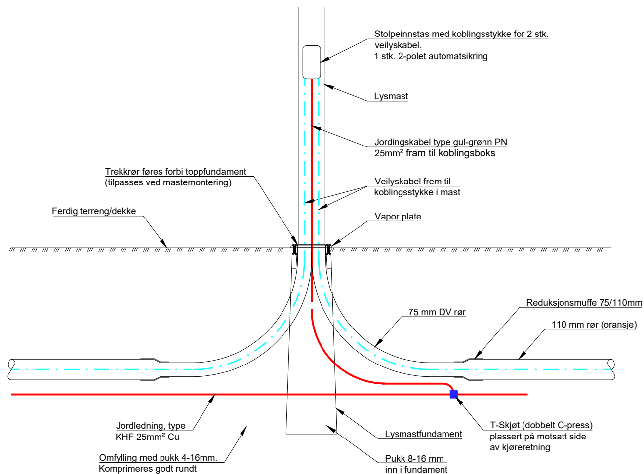
SNITT B-B
