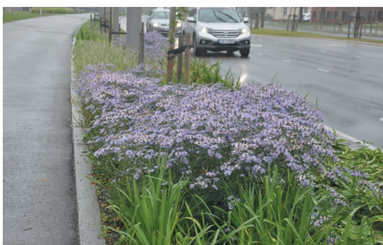
Figur 5-5: Eksempel på langsgående blågrønn løsning (nedsenket grøntrabatt/regnbed) i gate der overvannet fra veibane/GS-vei infiltreres og renses i rabatten. Bjørnstjerne Bjørnsons gate i Drammen, fotoet til høyre er tatt etter et kraftig regnvær (Foto: SVV/Ane Kirstine Laukli).
