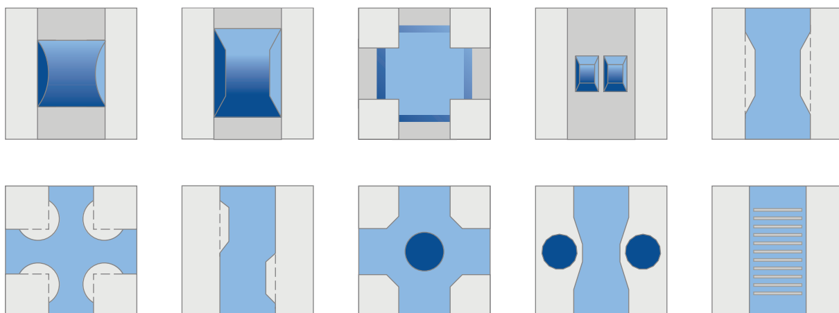
Figur 3-24: Ulike typer fartsreduserende tiltak (Statens vegvesens V128 Fartsdempende tiltak).
