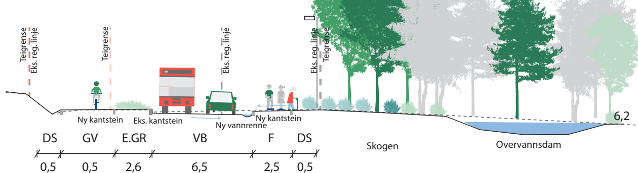
Oppriss 2 – Øst for ridesti
