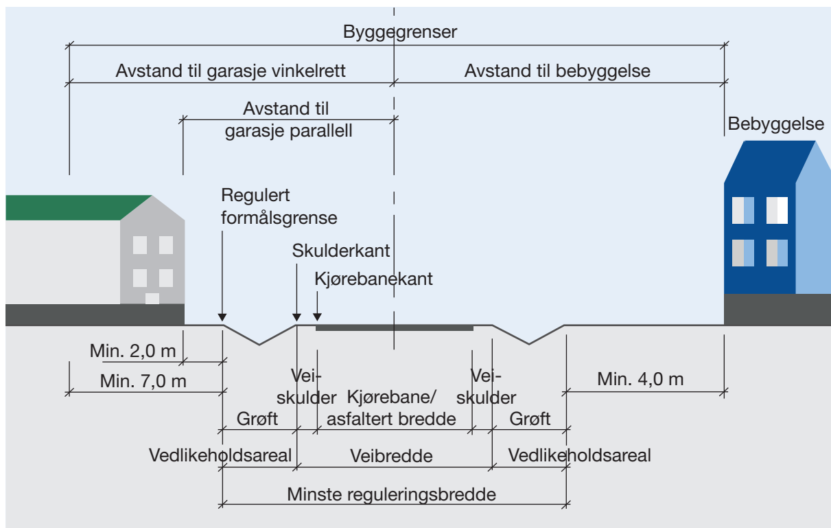
Figur 2-4: Veiens inndeling.
