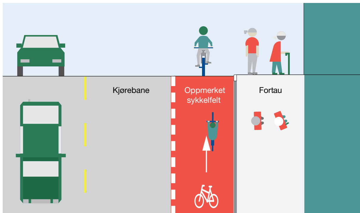
Figur 3-12: Oppmerket sykkelfelt.
