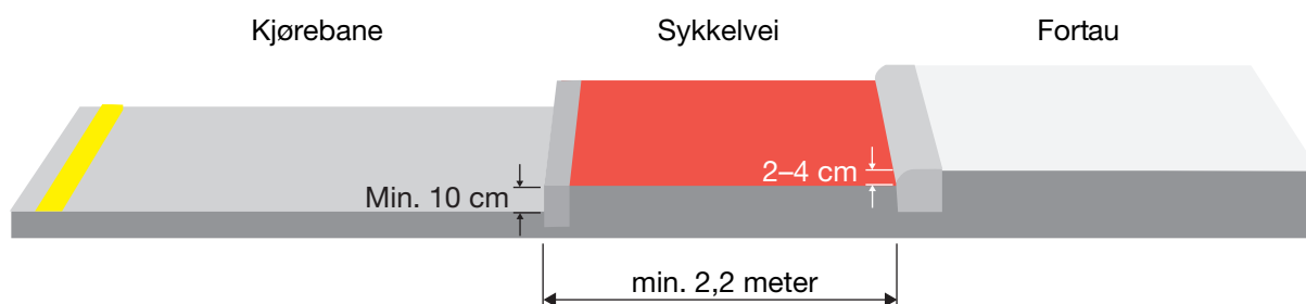
Figur 3-13: Standardmål for opphøyd sykkelfelt.
