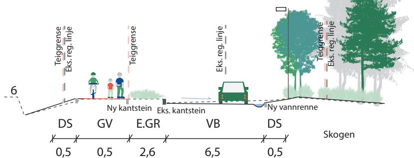
Oppriss – Vest for ridesti
