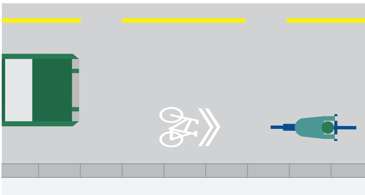
Figur 3-18: Delesymbol (Sharrows) i kjørebanelan.
