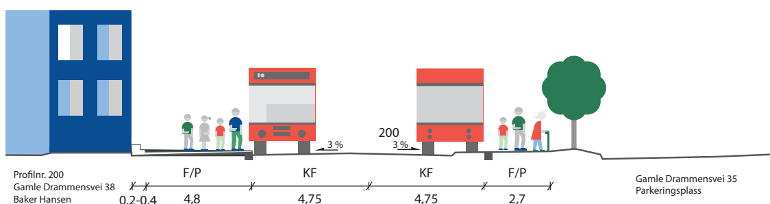
Tverrsnitt 13 meter
