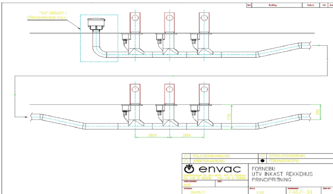
Figur 4: Eksempel på nedkast utvendig plassert.
